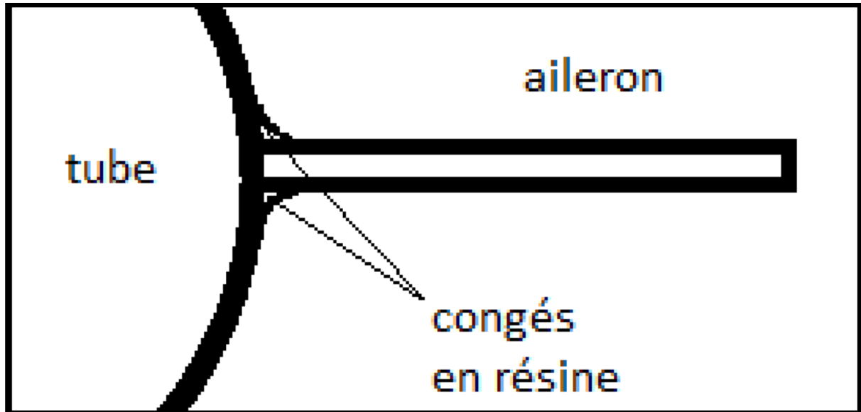
FIGURE 3.3 – Procédé de collage ailerons/structure avec congés en résine
