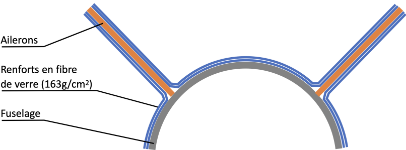
FIGURE 3.4 – Illustration du collage des ailerons sur le tube de la mini-fusée Arcturus .
