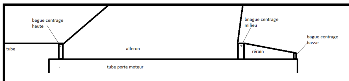
FIGURE 3.2 – Procédé de collage ailerons/tube porte-moteur
