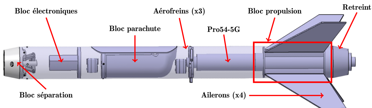
FIGURE 3.1 – Vue du premier étage sur CATIA
